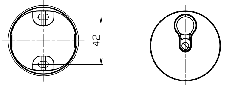
C-C断面図 (S=1:2)
